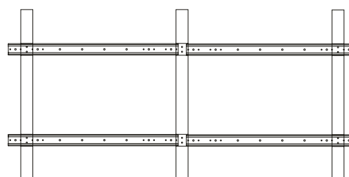
S615 | Dubbel för 8 Moduler | 4x2 Balk
