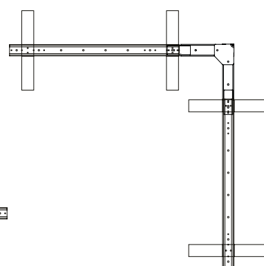
S616 | Hörn för 1 Modul | 1x1 Balk S614 | Singel för 4 Moduler | 2x2 Balk
