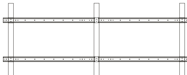
S615 | Dubbel för 10 Moduler | 4x2,5 Balk
