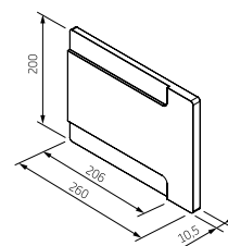
Stor monteringsplatta utan hål för tak eller vägg. Tak/Väggbeslaget skruvas fast i monteringsplattan
