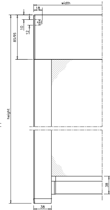
Kasset, sido- och underlist – motorutgång baktill
